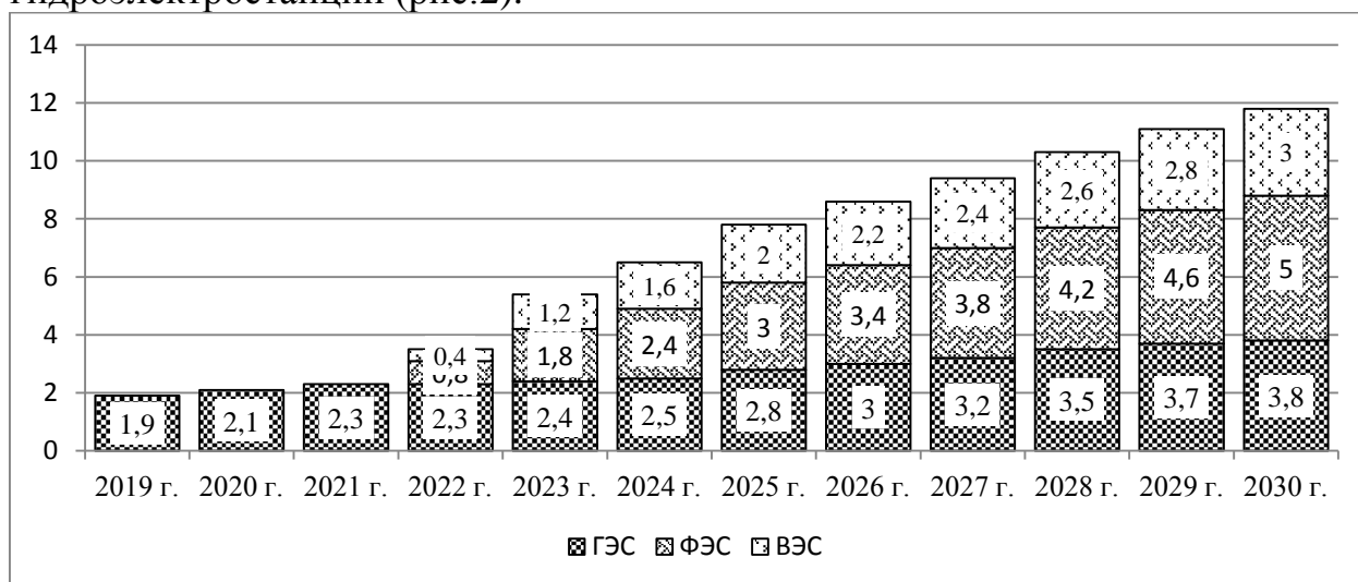
Рис. 2. Структура генерации Республики Узбекистан на основе возобновляемых источников энергии к 2030 г., МВт
