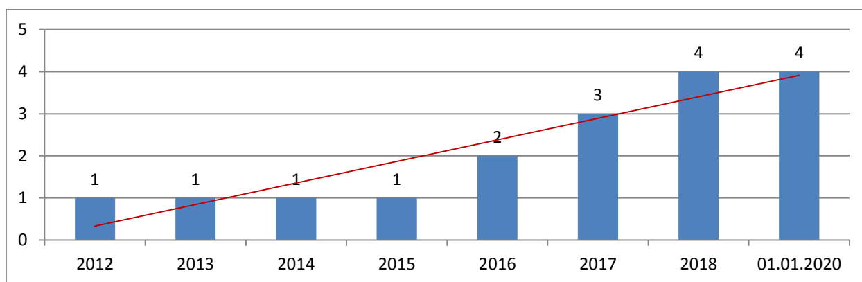
Рис. 3. Динамика мощности объектов солнечных электростанций в Узбекистане в период с 2012 по 2020 год, МВт [24]
