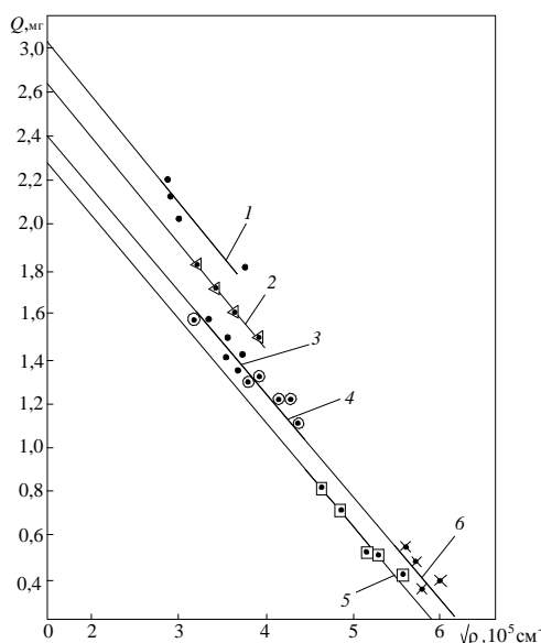
Рис. 1. Зависимости изменения износов Q образцов из низкоотпущенных сталей 30 (1), 45 (2), 30 без отпуска (3), 55 (4), У8 (5) и 65Г(6) от плотности \sqrt{\rho} дислокаций
