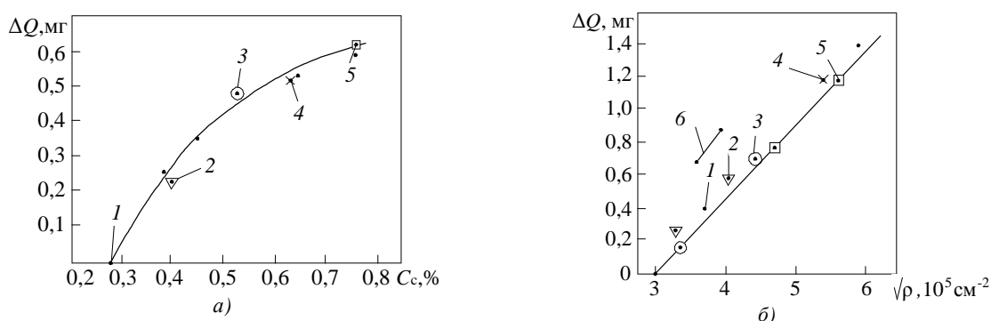
Рис. 2. Значения разниц \Delta Q износов для сталей 30 (1), 45 (2), 55 (3), 65Г (4), У8 (5) и стали 30 без отпуска (6) в зависимости от содержания C_c углерода в мартенсите (а) и от плотности \sqrt{\rho} дислокаций (б), а также их аппроксимирующие кривые
