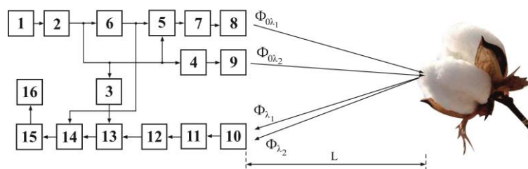
Рис.1. Блок схема устройства для дистанционного контроля влажности хлопка – сырца.
