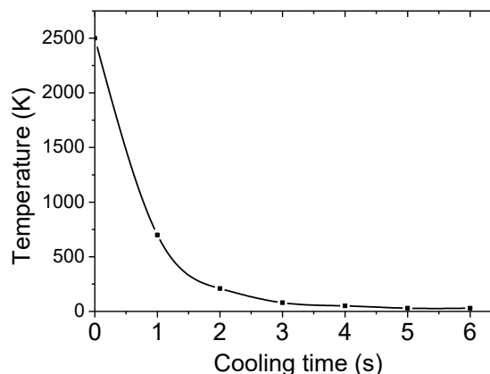
Рис.3. Кривая охлаждения расплава на солнечной печи методом слива капель жидкости в воду при \alpha=1000 Вт/(м 2 К).
