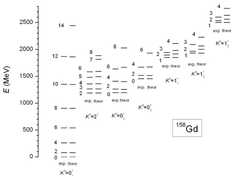
Рис.1. Сравнение спектров энергий состояний с положительной четностью в ^{158}\text{Gd} .
