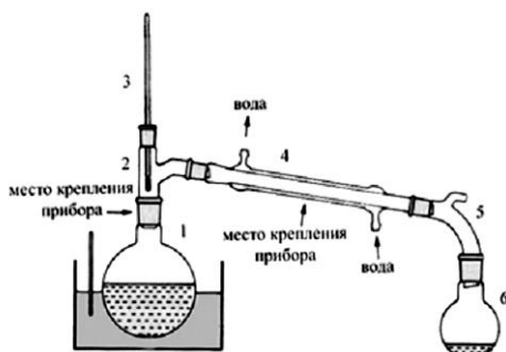
Рис. 1. Установка для простой перегонки: 1 - перегонная колба, 2 - насадка, 3 - термометр, 4 - холодильник, 5 - аллонж, 6 - приемная колба.
