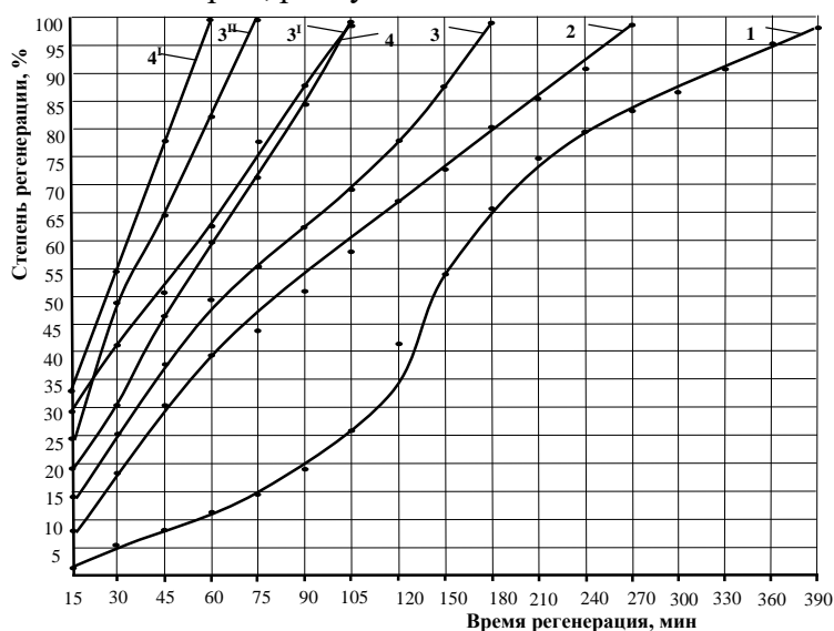
Рис. 3. Скорость регенерации этилового спирта из НАКР в зависимости от продолжительности перегонки, температуры и давления. Температура, °С: 1 (30); 2 (50); 3,3 I ,3 II (70); 4, 4 I (80); давление: 1–4(атм); 3 I (0,1 атм); 3 II ,4 I (0,3 атм).
