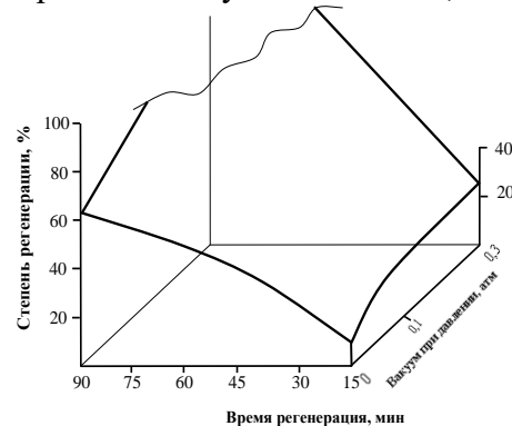
Рис. 4. Скорость регенерации этилового спирта из НАКР в зависимости от продолжительности и давления перегонки при температуре 70°C.
