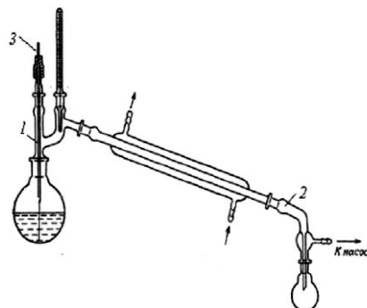
Рис. 2. Установка для вакуумной Перегонки: 1 - насадка; 2 - аллонж; 3 - капилляр.
