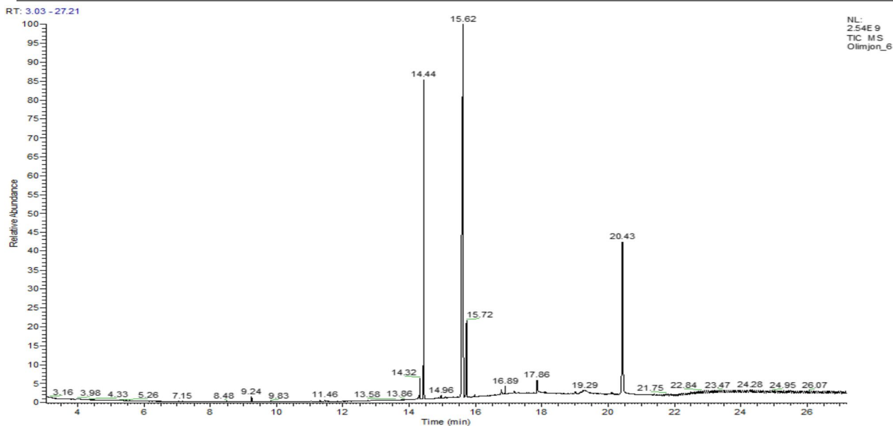
Рисунок 2. Хроматограмма метиловых эфиров жирных кислот оливкового масла.
