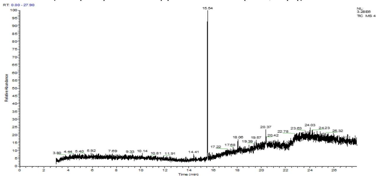
Рисунок 7. Хроматограмма метиловых эфиров рафинированного подсолнечного масла. Видно, что состав подсолнечного масла состоит в основном из ненасыщенных жирных кислот.
