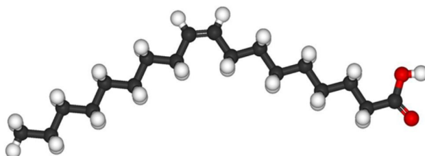
Рисунок 1. Структура олеиновой кислоты.
