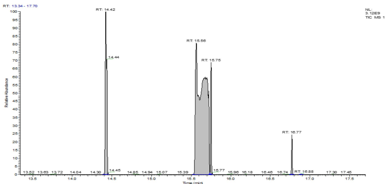
Рисунок 4. Хроматограмма метиловых эфиров олеиновой кислоты, полученная из рапсового масла методом метилирования.
