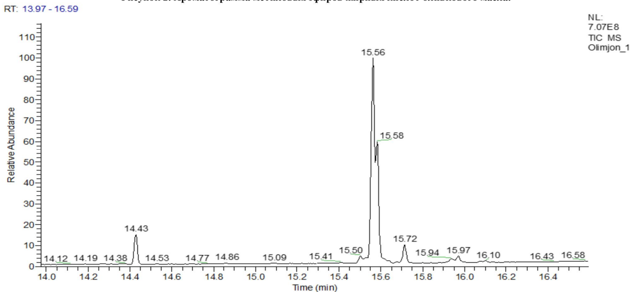
Рисунок 3. Хроматограмма метиловых эфиров жирных кислот подсолнечного масла.
