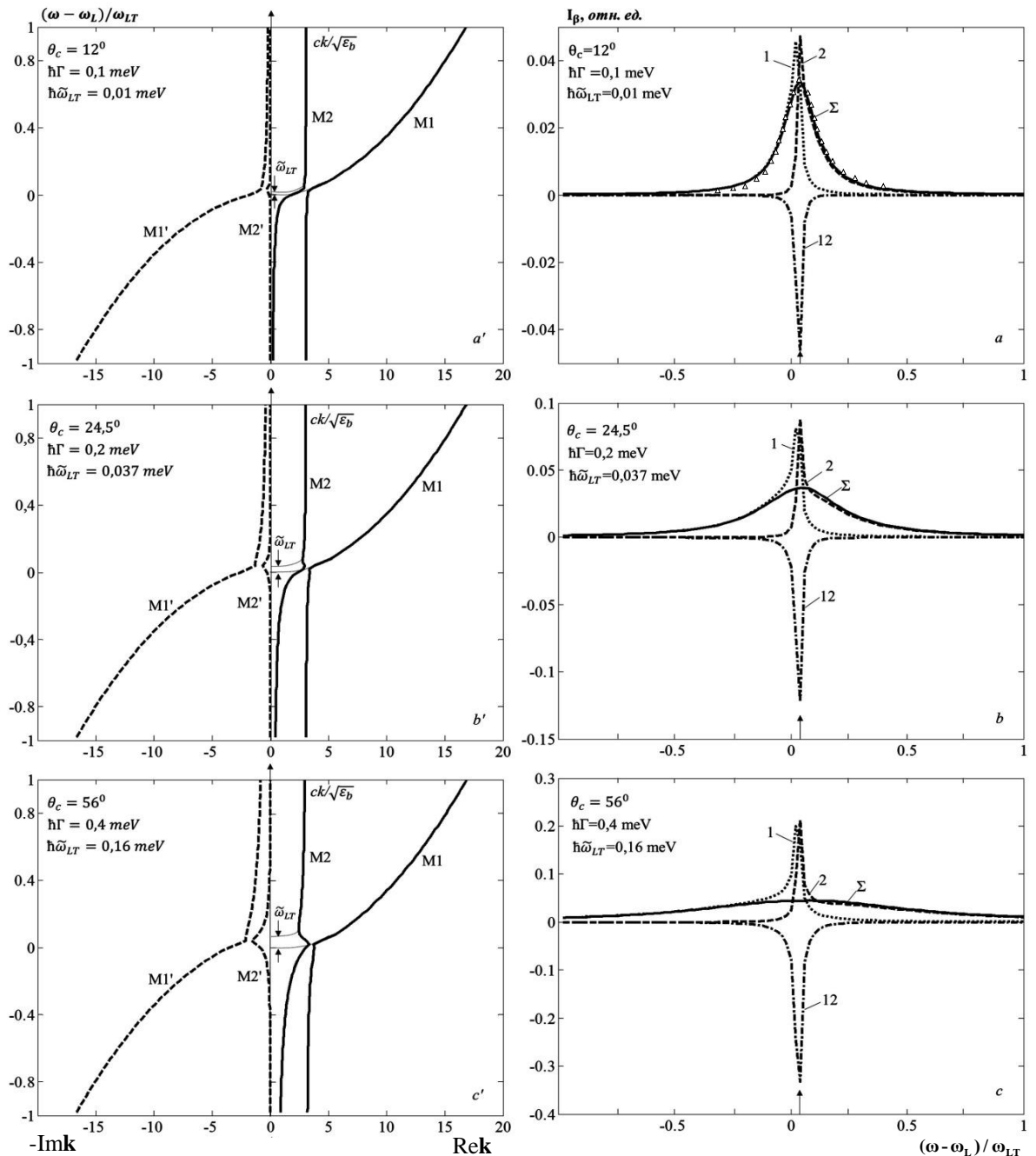
Рис.2. Сравнение дисперсионных кривых ( a'-c' ) и спектров фотолуминесценции ( a-c ) смешанных мод при критических значениях \Gamma_c = \Gamma , рассчитанных для значений параметров CdS при T=2 К. Треугольники-
