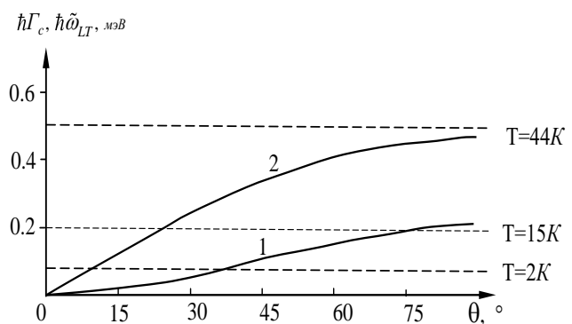
Рис. 1. Зависимости от угла выхода \theta значений \tilde{\omega}_{LT} (1) и \Gamma_c (2), рассчитанные для параметров смешанных мод экситонного резонанса A_{n=1} в CdS .
