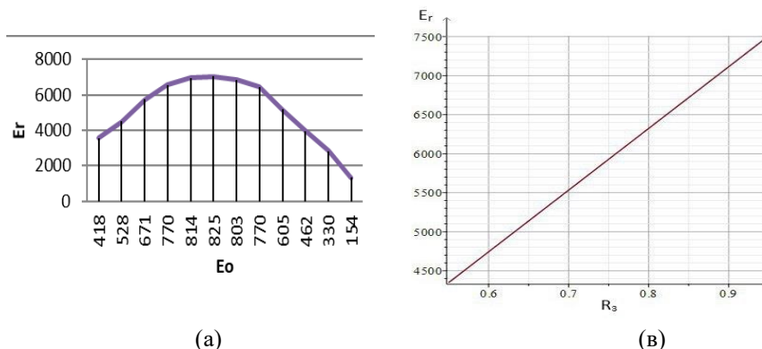
Рис. 2. Влияние параметра E_0 , (а) и R_3 , (в) на плотность потока солнечного излучения.
