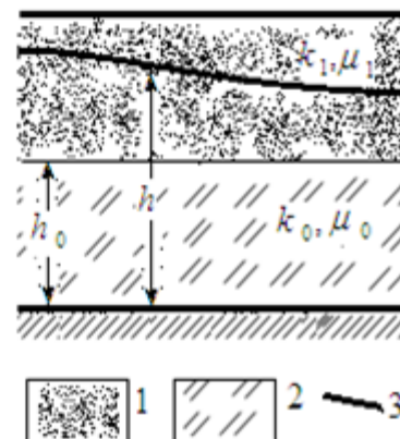
Рис. 2. Схема неоднородного строения водоносного пласта. 1-песок. 2-суглесь или глинистый песок. 3-зеркало грунтовых вод.
