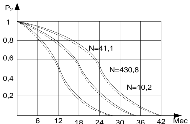
Рис. 2. Зависимость вероятности безотказной работы от сработанного ресурса; (сплошными кривыми при неравномерном и штриховыми - при равномерном износе).
