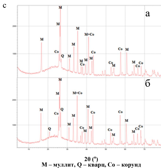
Рисунок 6. Дифрактограмма глинистого сланца с добавкой 20% \text{Al}_2\text{O}_3 , обожженных при 1300 °C (а), 1400 °C (б).
