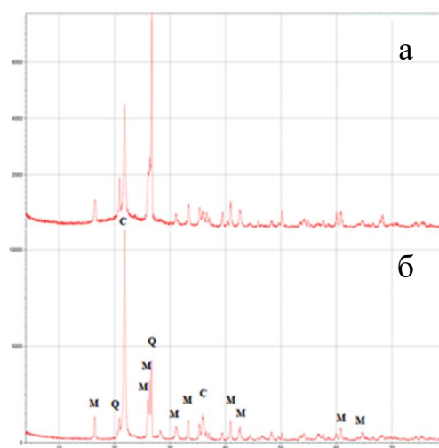
С – кристобалит, М – муллит, Q – кварц
