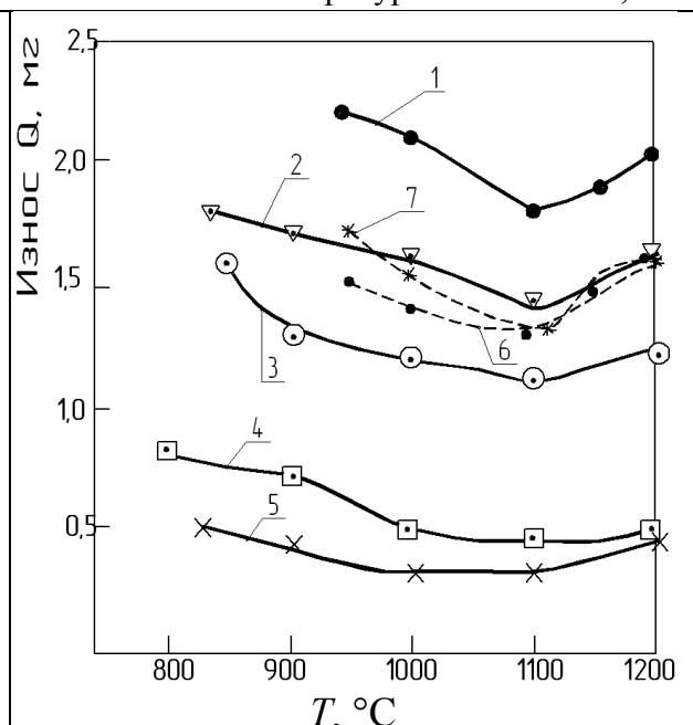
Рис. 3. Влияние температуры T предварительной нормализации на износ Q после повторной закалки и отпуска при 200 °С для сталей Ст5Гпс (1), 35 (2), 45 (3), У8 (4), 65Г (5) и стали Ст5Гпс без отпуска (6 и 7, где 7-непосредственная закалка с указанных температур).
