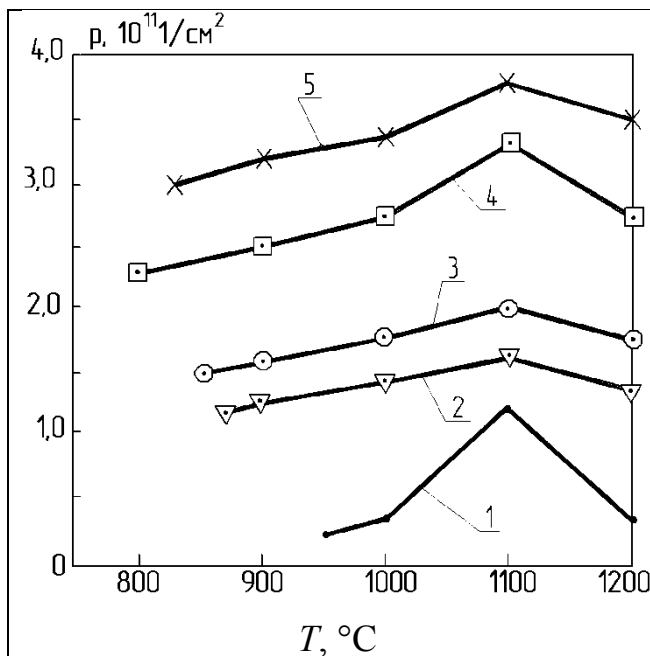
Рис. 2. Влияние температуры T предварительной нормализации на плотность \rho дислокаций после повторной закалки с температуры нагрева A_{c3} + (30 \div 50) °С (стали Ст5Гпс, 35, 45, 65Г) и A_{c1} + (30 \div 50) °С (сталь У8) и отпуска при 200 °С; стали: Ст5Гпс (1), 35 (2), 45 (3), 65Г (4) и У8 (5).
