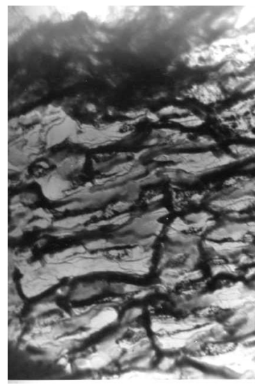
в) Микрофотографии (хэ3200) скола цементного камня оптимального состава (образцы 28 сут. возраста)
