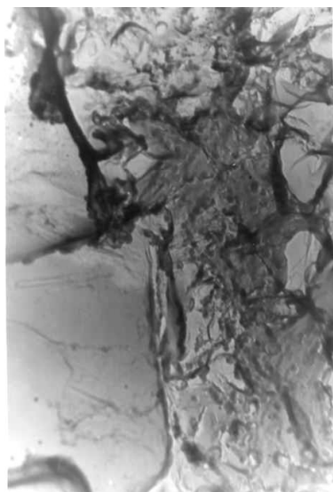
Рис.3. а) Микрофотографии (хэ3200) скола цементного камня не оптимального состава - с избытком воды (образцы 28 сут. возраста)
