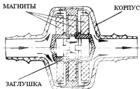
Рис.1. Схема конструкции устройства для магнитной обработки воды CO-2, CO-3.
