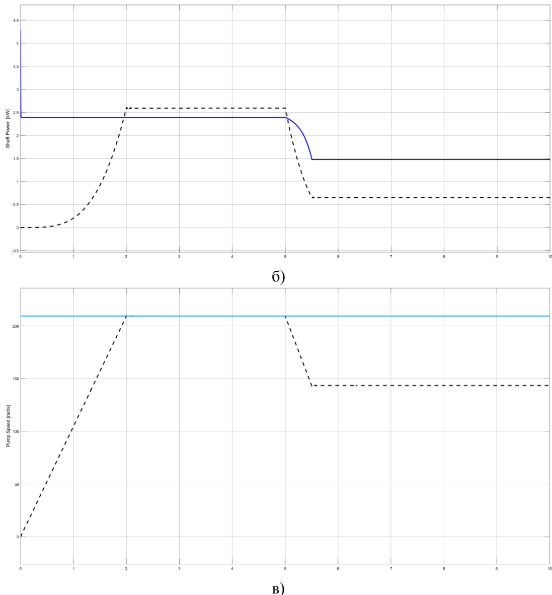
Рис. 3. Режим работы скважинной насосной установки при частотном регулировании скорости вращения (-----) и без регулирования скорости вращения ( _____ ): а) зависимость производительности от времени; б) зависимость мощности от времени; в) зависимость скорости вращения от времени.
