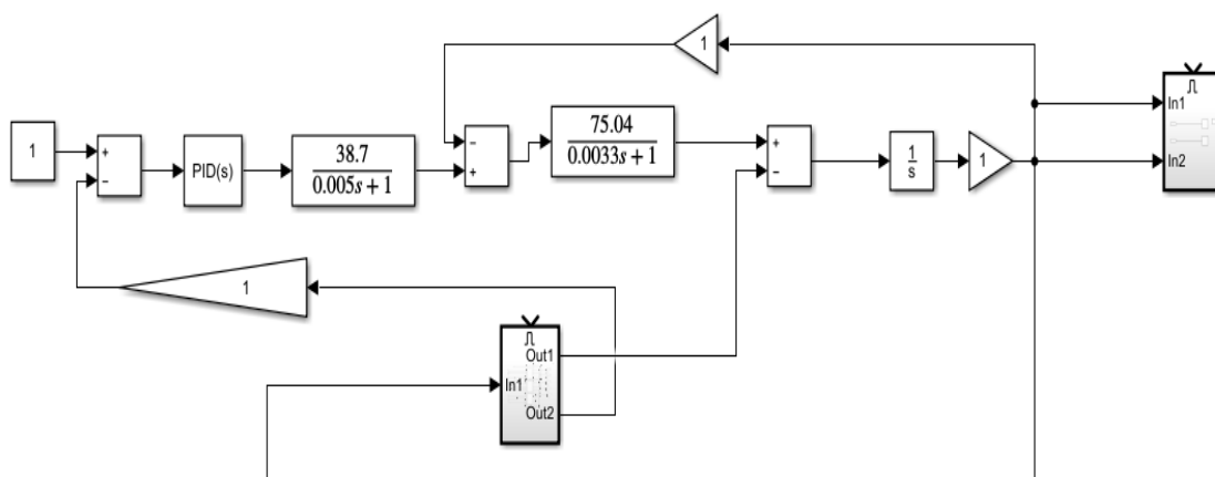
Рис. 2. Структурная схема частотно-регулируемого электропривода насосной установки.
