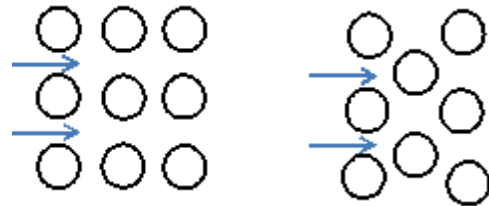
рис 2. Схема расположения трубок в калорифере а)-коридорная б) шахматная.
