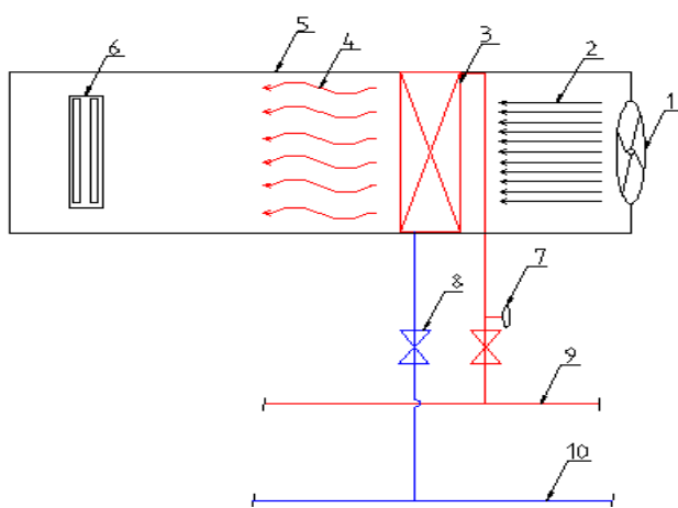
Рис.1. 1-вентилятор, 2-поток воздуха, 3-отопительный радиатор, 4-нагретый воздушный поток, 5-вентиляционная шахта, 6-диффузор, 7-термометр, 8-задвижки, 9-подача горячей воды.10- обратный поток воды.
