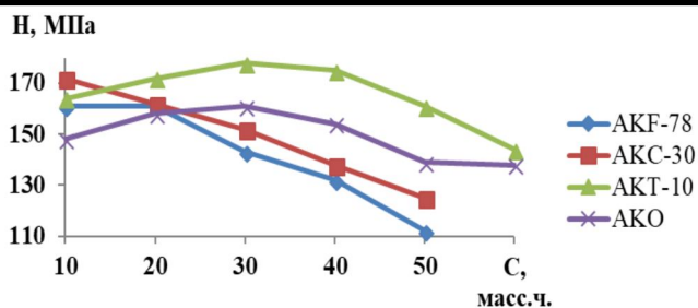
Рис. 1. Влияние вида и содержания наполнителей на микротвёрдость (H) эпоксидных покрытий.
