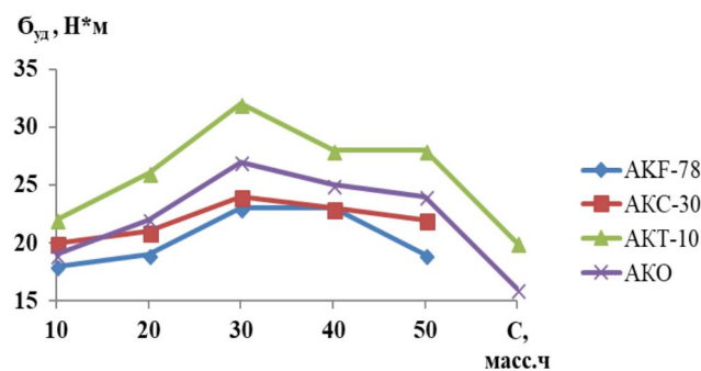
Рис. 2. Влияние вида и содержания наполнителей на ударную прочность (Bуд) эпоксидных покрытий.
