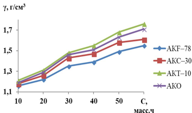
Рис. 3. Влияние вида и содержания наполнителей на плотность ( \gamma ) композитных эпоксидных покрытий
