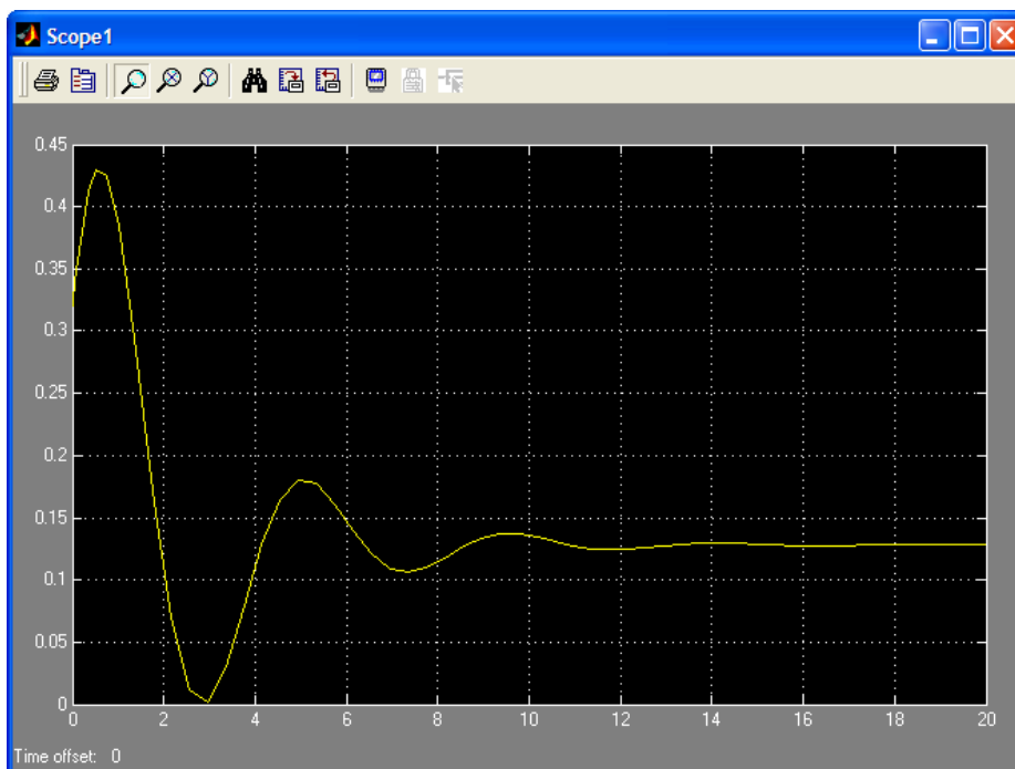
Рис.5. График процесса регулирования оптимального смешения.
