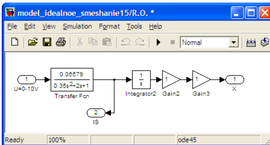
Рис.4. Схема подсистемы регулирующего органа (R.O.).
