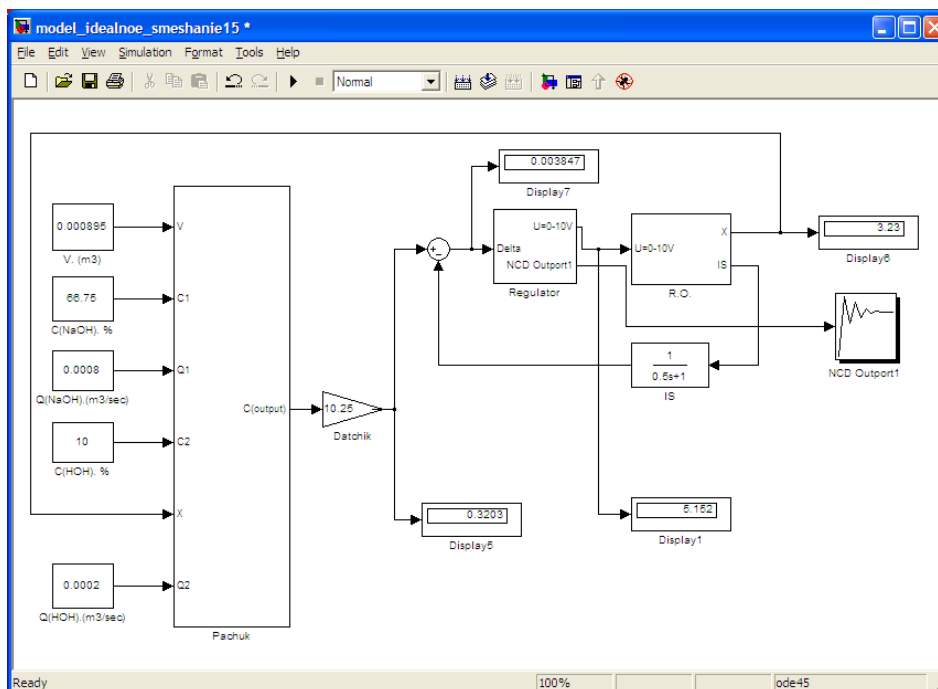
Рис.2. Схема математической модели.
