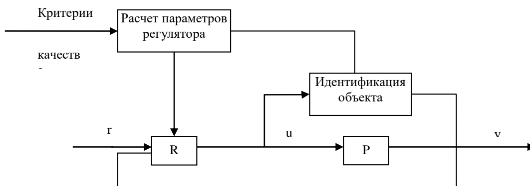
Рис. 1. Структурная схема автоматической системы управления.
